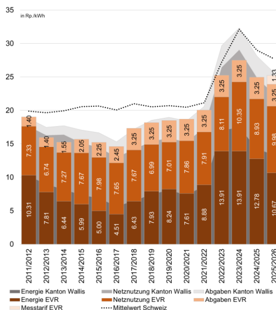
Strompreisentwicklung (H4) 2011/2012-2025/2026 EVR Energieversorgung Raron AG, Kanton Wallis und Schweiz (Quelle: Eidgenössische Elektrizitätskommission EICom)
